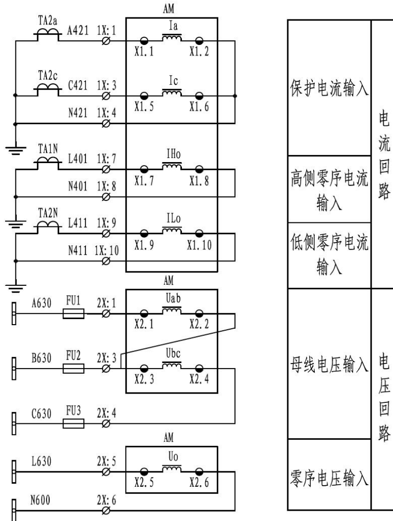
图 5.2 2PT 2CT 接线方法
